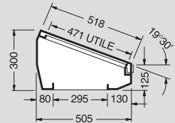
Alzata standard solo per base profonda 400 mm
