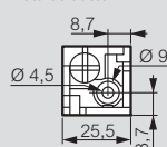
Vista da sotto
