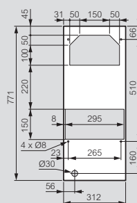
Art. 0 353 72/73
