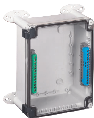
0 359 61 con staffe art. 0 358 02 e morsettiere IP2x
