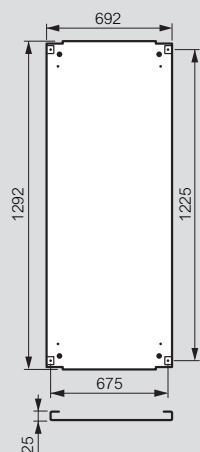
Piastra piena art. 0 349 59
