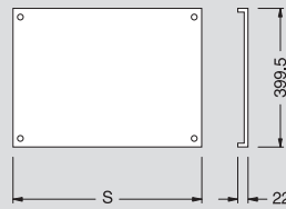
Piastra interna base
