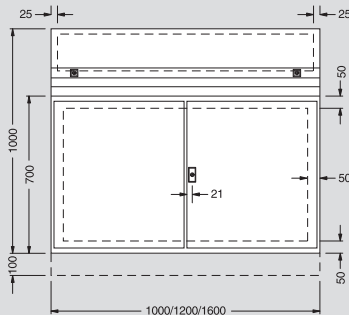
Alzatina per leggio compatto
