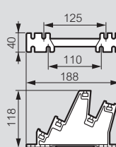
Art. 0 374 32
