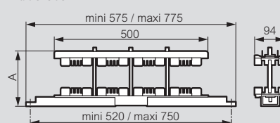
Art. 0 373 93
