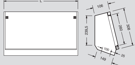
Alzatina per leggio compatto
