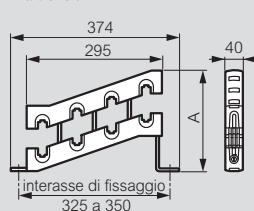
Art. 0 373 91
